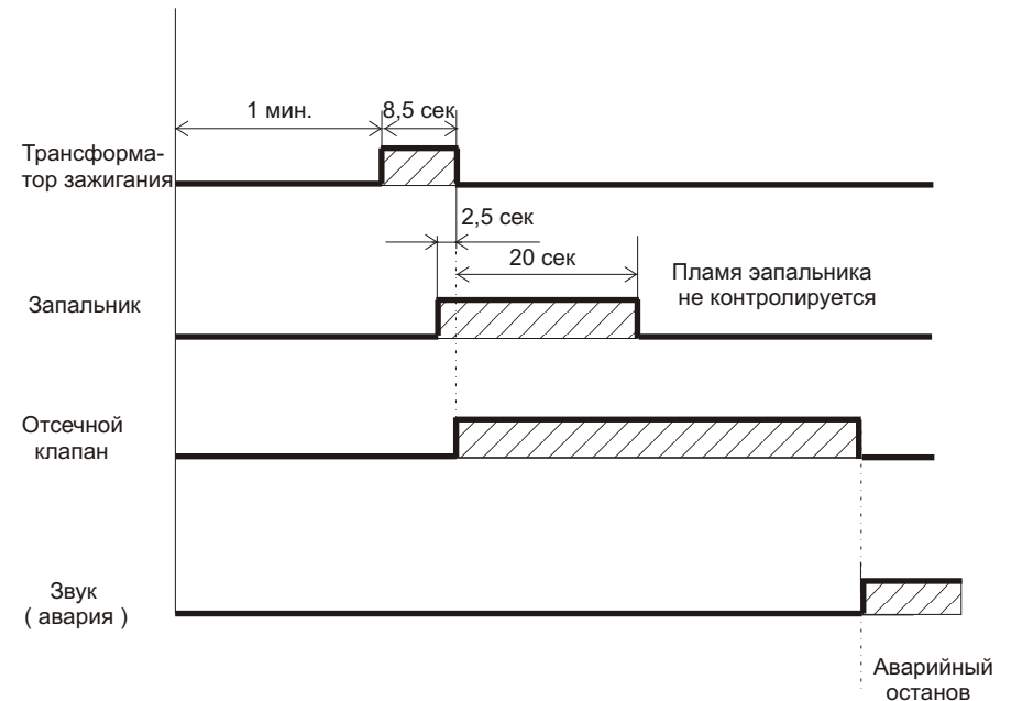
Временная диаграмма работы блока БУК-5МУПР
