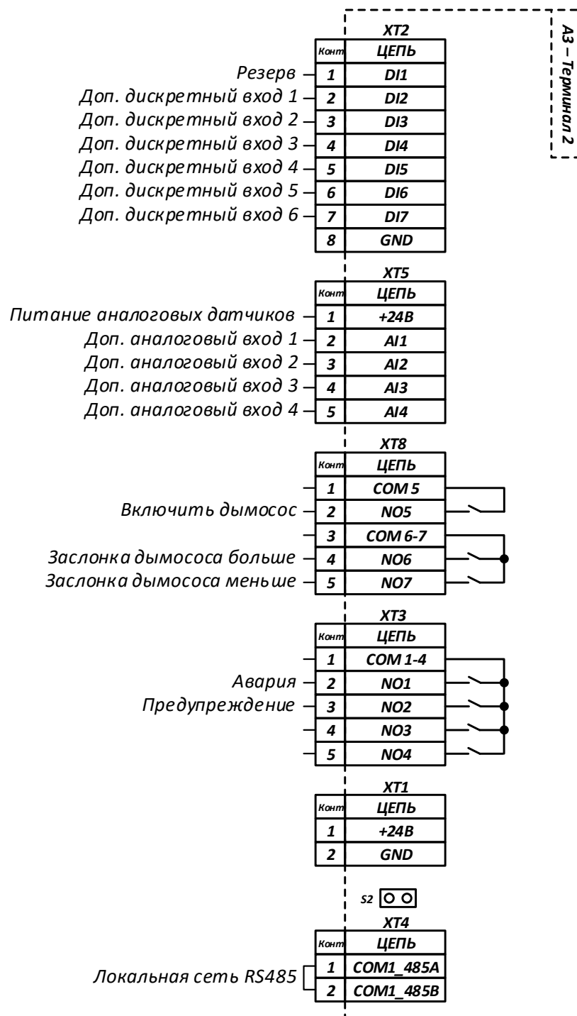
Рис. 5: А3 — Клеммы терминального блока 2.
