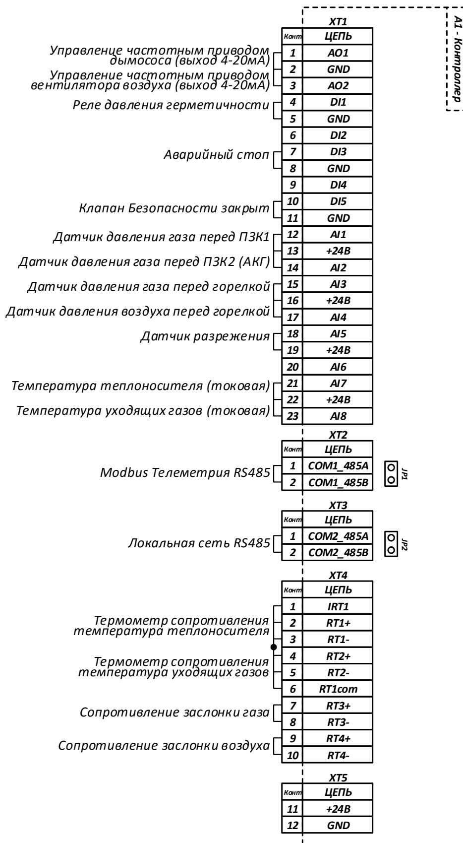
Рис. 1: А1 — Клеммы контроллера.
